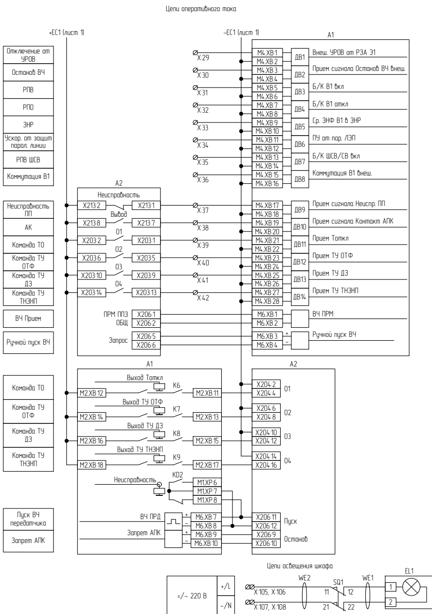
Рисунок В.2 – Схема электрическая принципиальная (часть 2)
