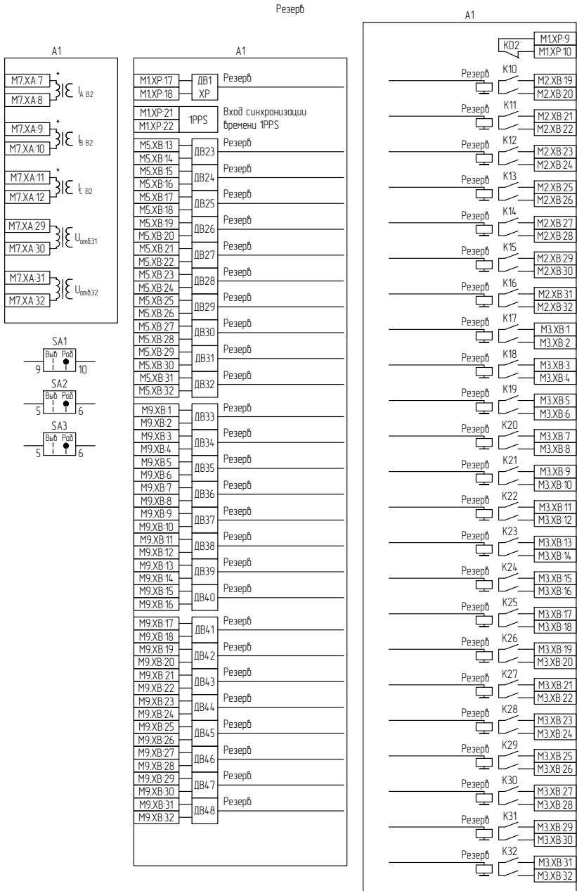
Рисунок В.3 – Схема электрическая принципиальная (часть 3)
